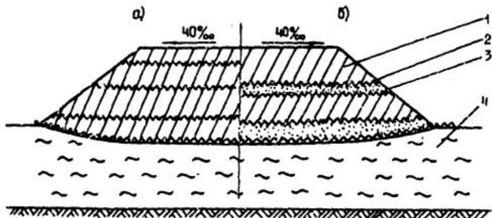
Рис. 4. Конструкции, насыпей с дренирующими прослойками из НСМ (а) или из песка с фильтром из НСМ (б):
