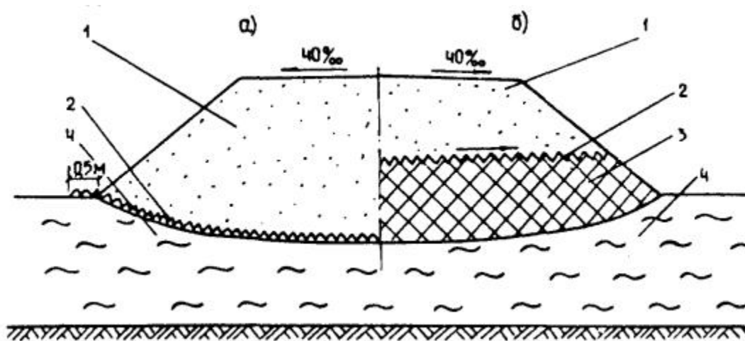
Рис. 1. Конструкция насыпи на слабом грунте с прослойкой из НСМ в основании насыпи (а) или над нижней частью насыпи из местного грунта (б):
