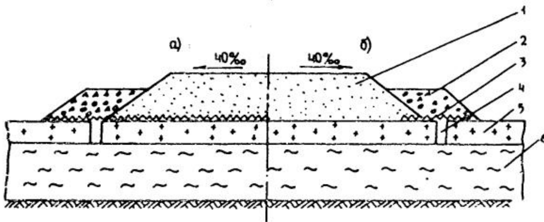
Рис. 3. Конструкция насыпи с прорезями, перекрытыми прослойкой из НСМ, проложенной либо на всю ширину насыпи (а), либо над прорезями (б) с выпуском за пределы прорези не менее чем на три ее ширины:
