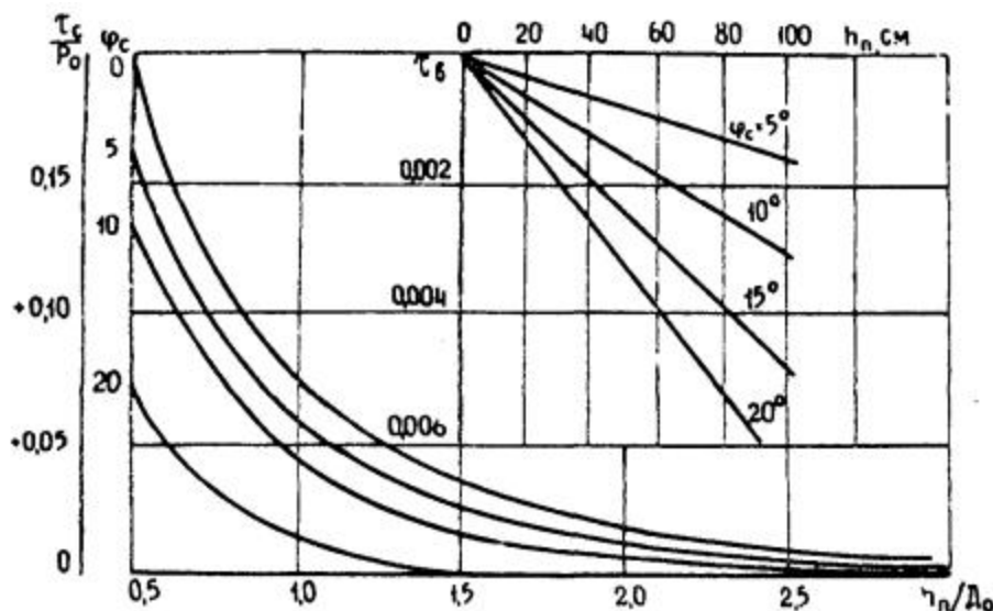
Рис. 12. Зависимость относительного активного сдвигающего напряжения t_c/p_0 и поправки на собственный вес грунта t_b от толщины песчаного слоя h_n
