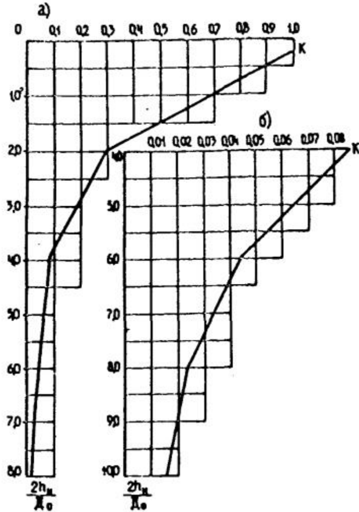
Рис. 10. Зависимость коэффициента распределения напряжений K_p от относительной координаты глубины
