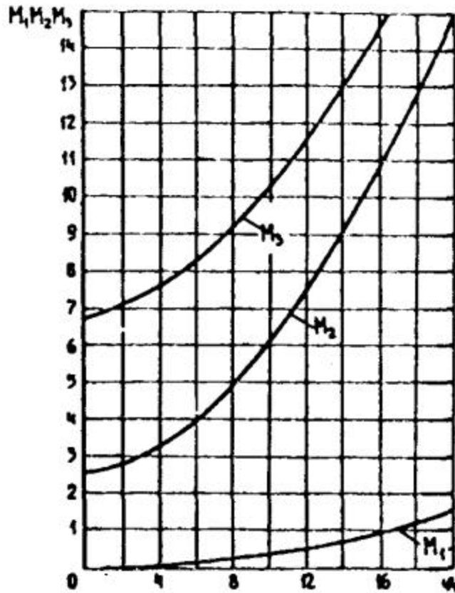
Рис. 11. Зависимость коэффициентов M_1 , M_2 , M_3 от угла внутреннего трения слабого грунта \phi_c
