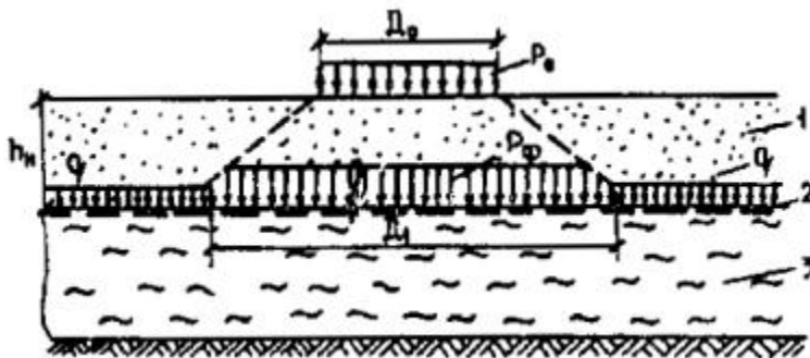
Рис. 9. Схема расчета толщины насыпи h_n с прослойкой из НСМ, обеспечивающей допустимую глубину колеи по условию движения:
