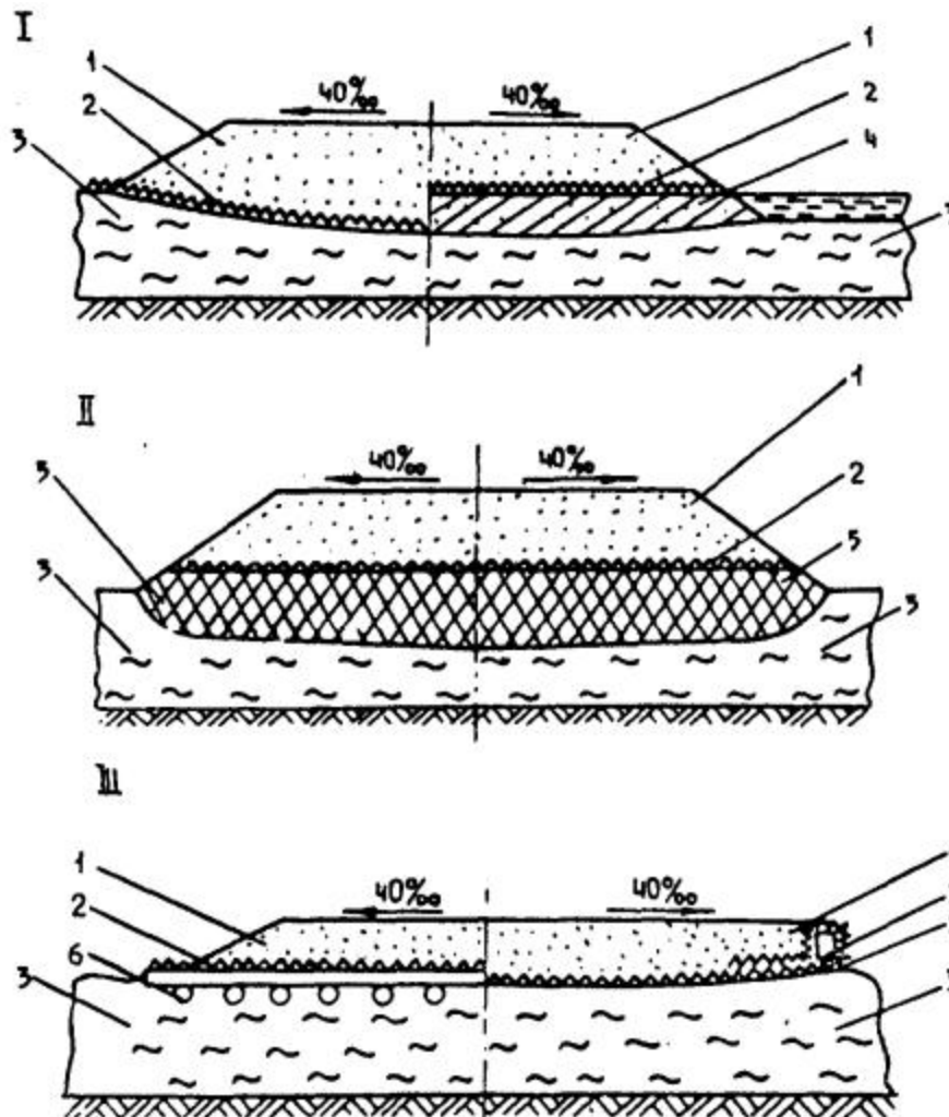
Рис. 8. Три типа конструкций насыпей (I, II, III) временных дорог с прослойкой из НСМ:
