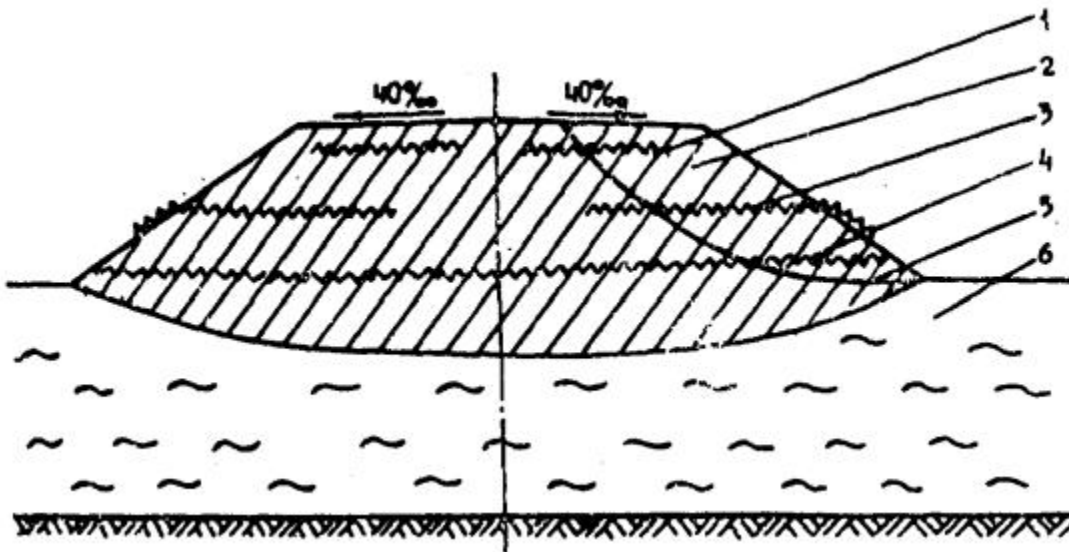
Рис. 6. Армирование насыпи прослойками из НСМ:
