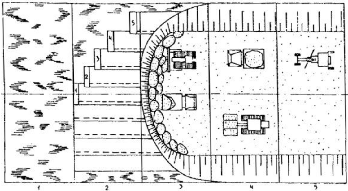
Рис. 13. Технологическая схема устройства прослоек из НСМ:
