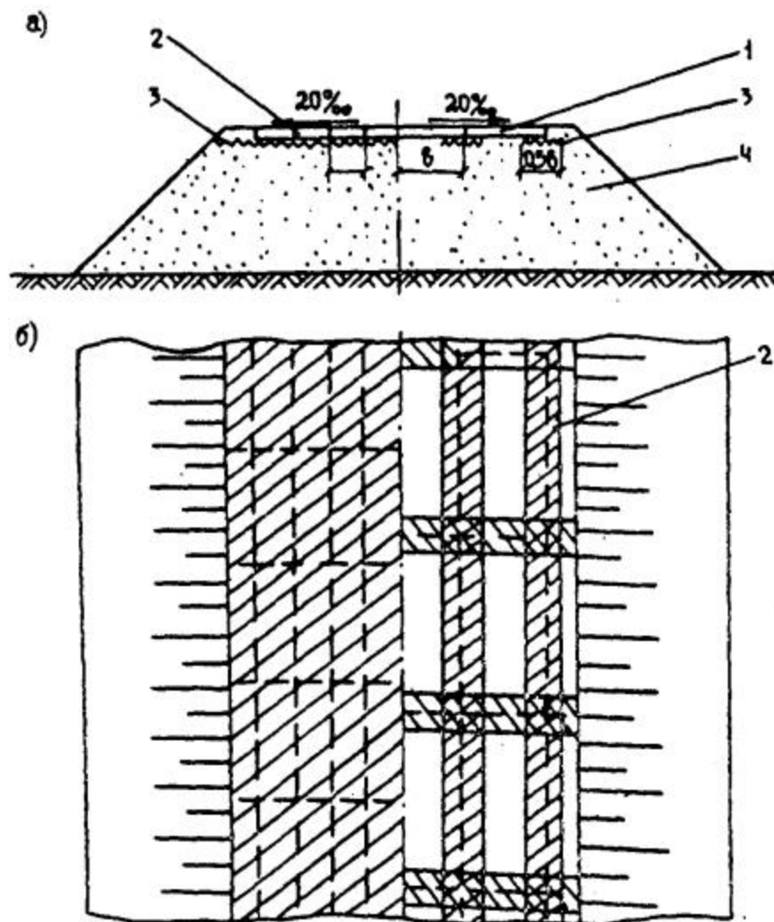
Рис. 7. Прослойка из НСМ в основании сборного покрытия в разрезе (а) и плане (б):
