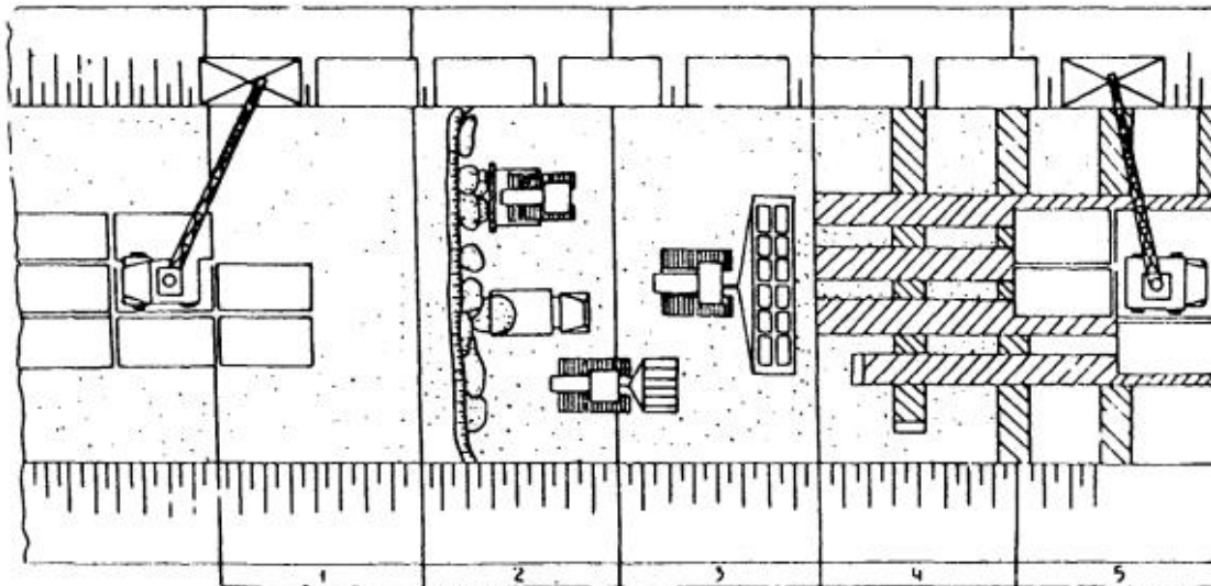
Рис. 14. Технологическая схема устройства прослоек из НСМ под сборным покрытием:
